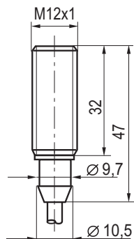
Габаритный чертеж
